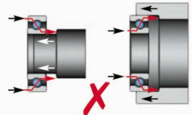
錯誤選用吸震墊圈將損傷軸承
