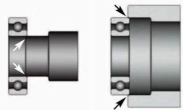
軸的過盈配合
